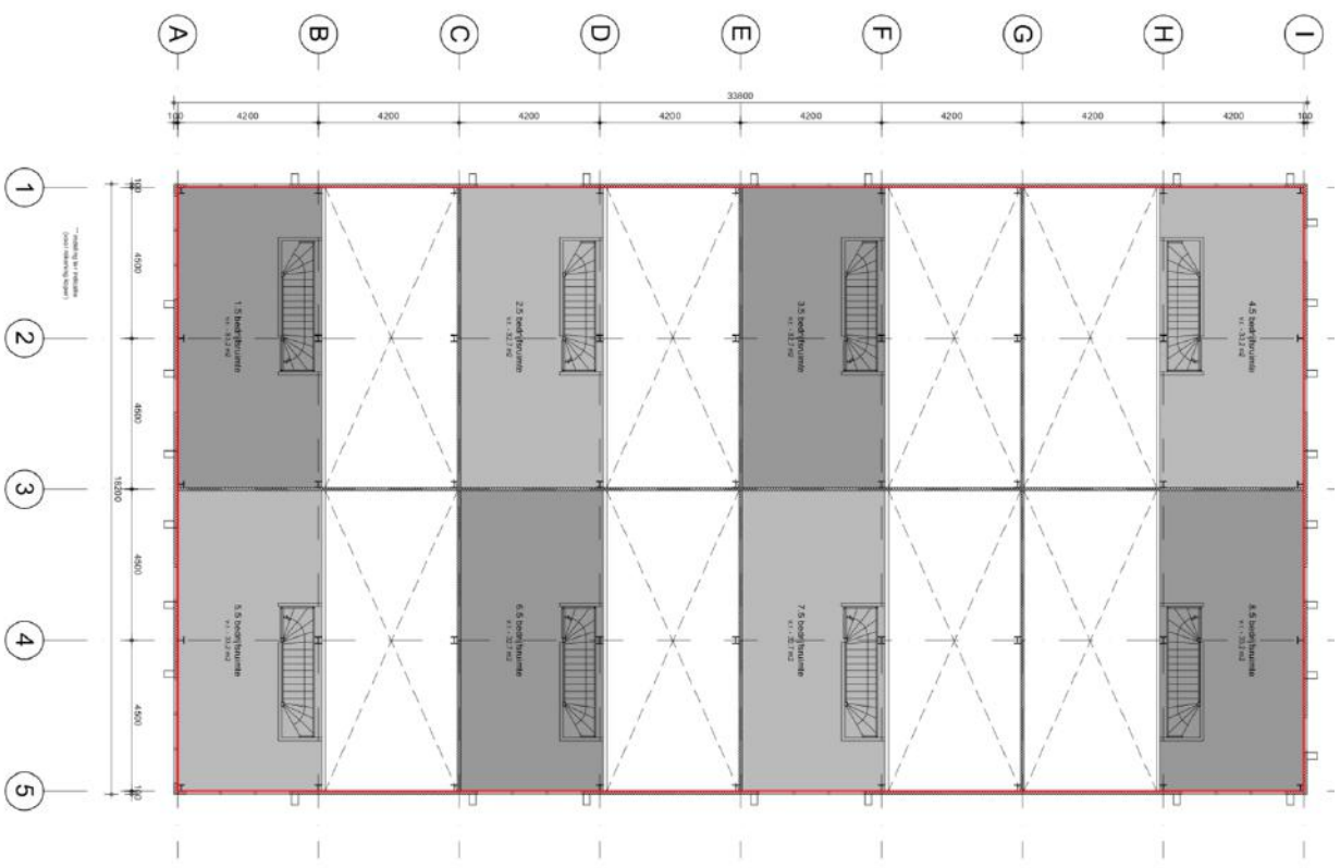
Plattegrond - 1e Verdieping (3500+ P.)
