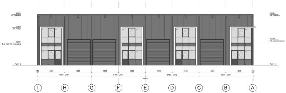
Aanzicht - Linker Zijgevel (noord-west)
